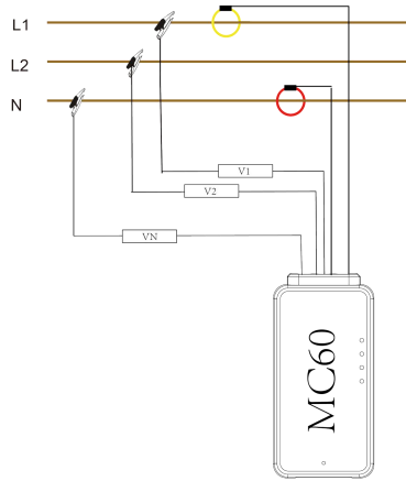
3P3W_2CT
